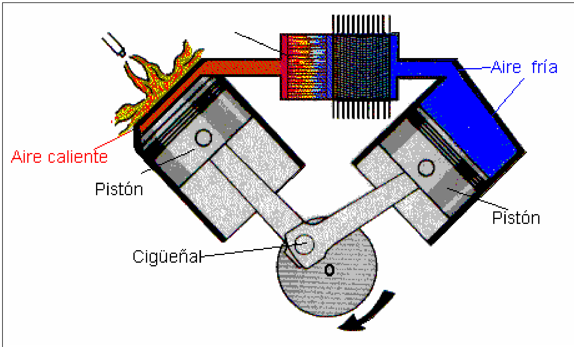
MOTOR DE STIRLING
